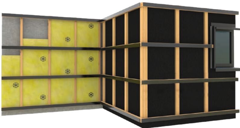
Konstruktion ohne Fassadenbahn
